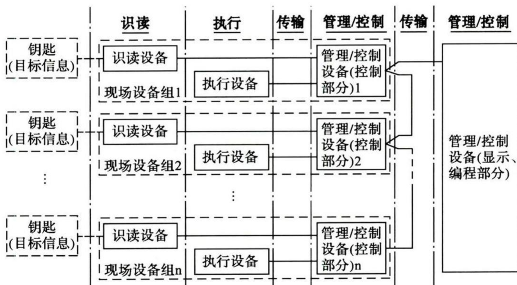
图 4.0.5-1 总线制系统组成
