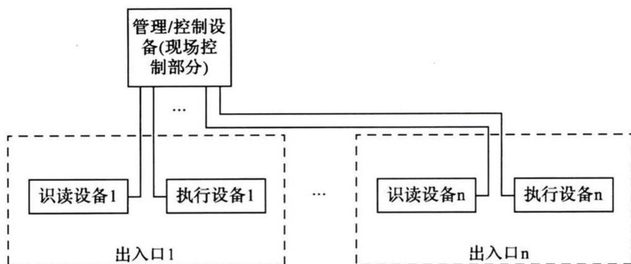
图 4.0.4-2 多出入口控制设备型组成
