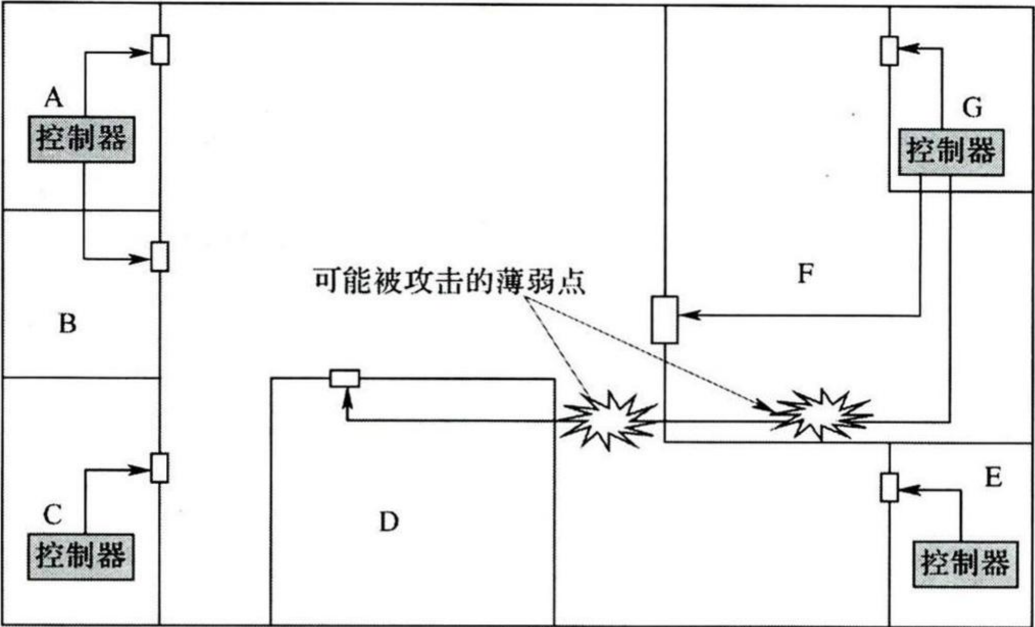
图 8 电控锁连线的布设对安全的影响
